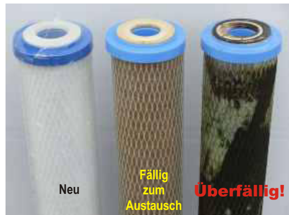
Abb.2: Aktivkohleblock-Filter 10µ.
